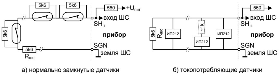
Рисунок 8 – Примеры монтажа пожарных шлейфов
