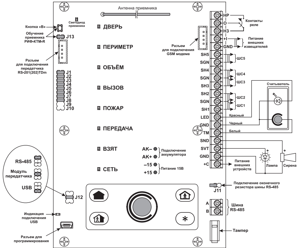
Рисунок 12 – Монтажная схема прибора
