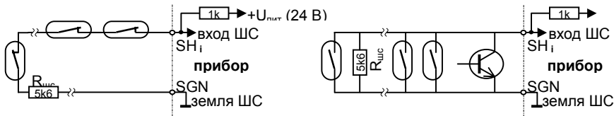
а) нормально замкнутые датчики
